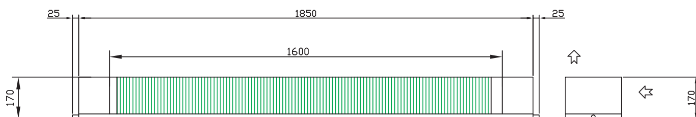
VISTA FRONTALE
