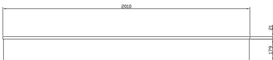
VISTA FRONTALE
