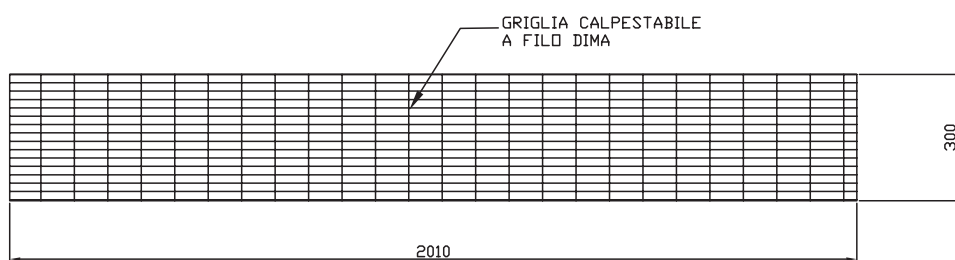
VISTA FRONTALE
