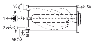
Serie A/VA mod. 80 ÷ 100x2/AU
