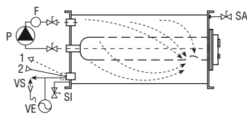
Serie A/VA mod. 130x2 ÷ 400x2/AP
